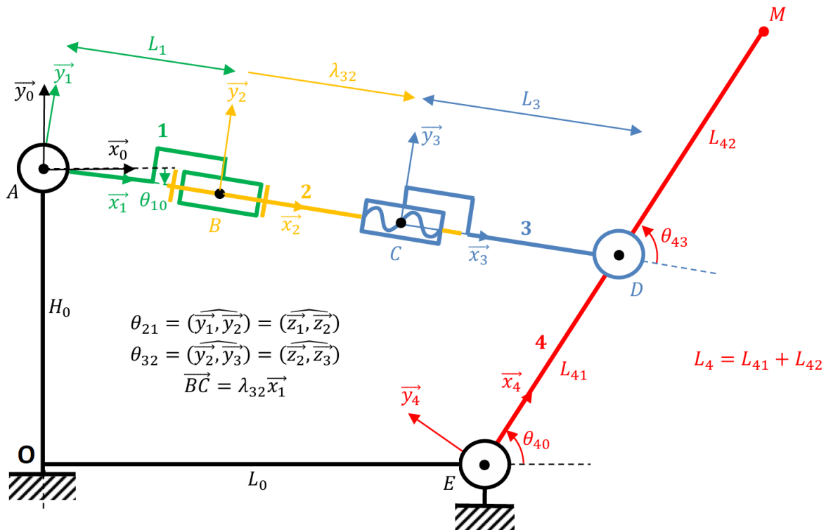
Schéma Cinématique de la maquette
